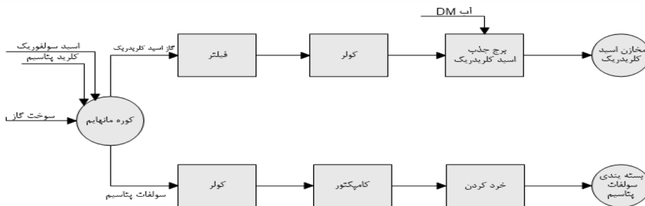
نمودار فرآیند تولید سولفات پتاسیم
